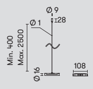
71-8262-05-05 ■ Linear connector - Conector lineal - Connecteur linéaire
