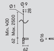
71-8260-05-05 ■ 90° vertical connector - Conector 90° vertical - Connecteur 90° vertical
